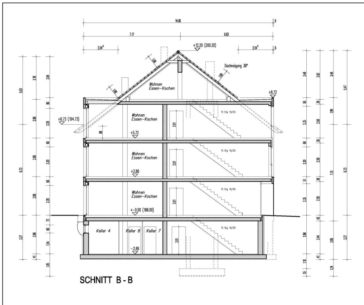
Abb.11: Gebäudeschnitt, unmaßstäblich
