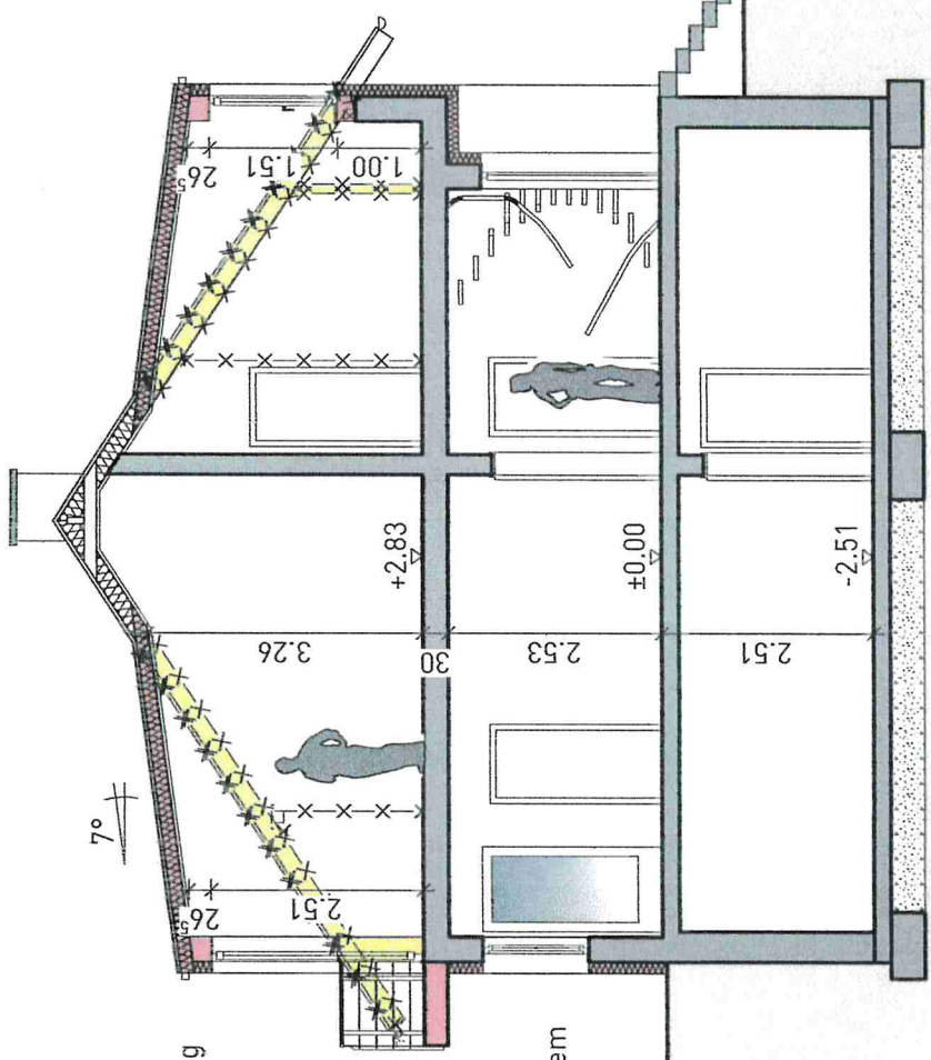
SCHNITT A-A
